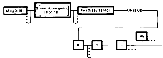
(d) C.mmp CMU multi-miniprocessor computer structure.
